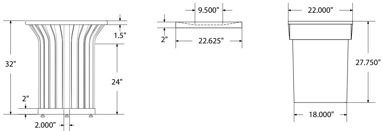
RECEPTACLE
