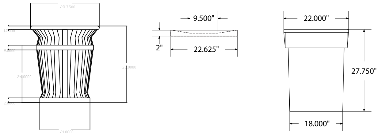
RECEPTACLE
